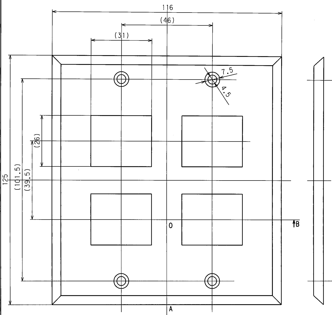
A-O-B断面図
