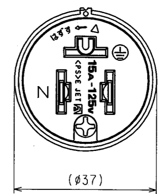
さし込みプラグ正面図
