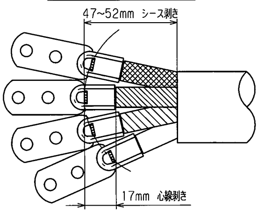
電線加工寸法 (参考値) 1/2
