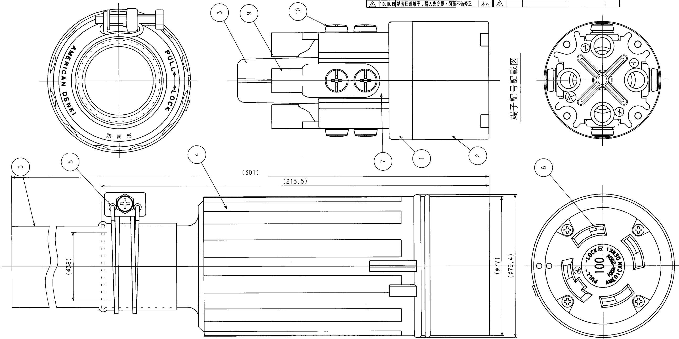
電線加工寸法 (参考値) 1/2
