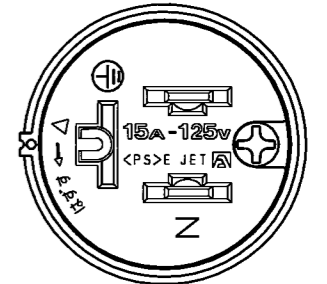
さし込みプラグ正面1/1図
