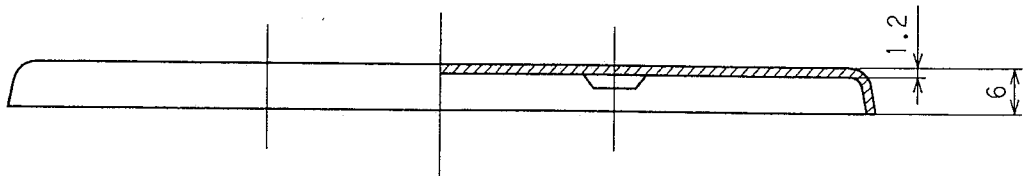
A-0-B断面図
