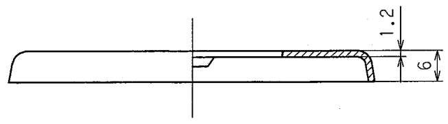
A-O-B断面図
