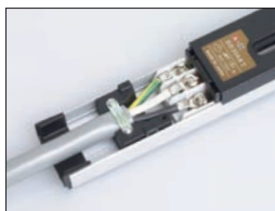
0Uコンセントバーとの接続例
