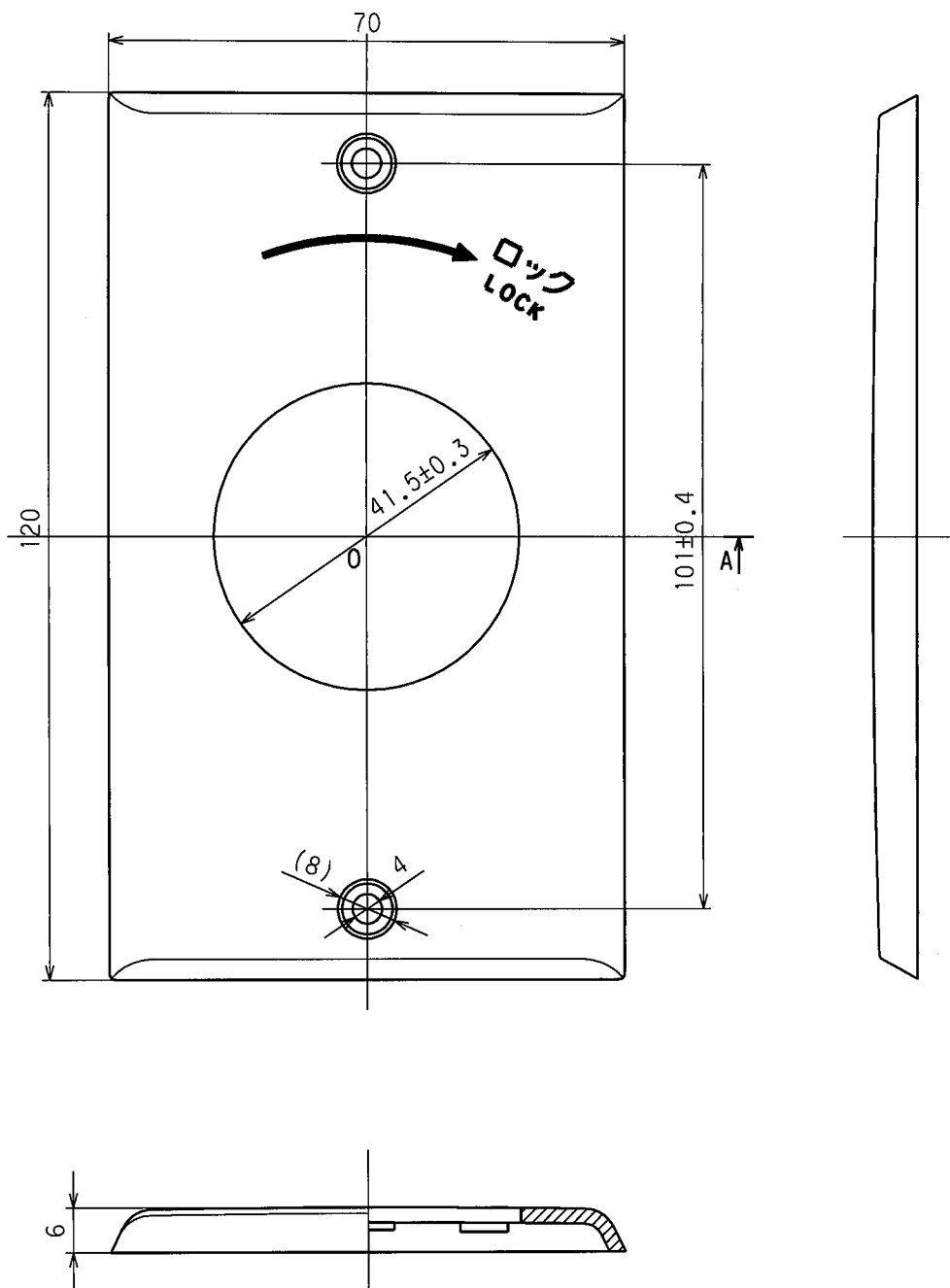
O-A断面
