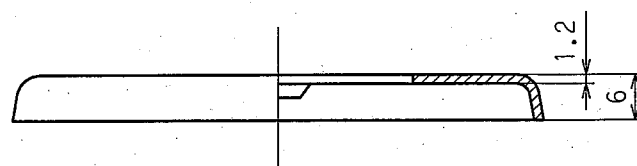
A-A断面図
