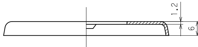
A-0-B断面図
