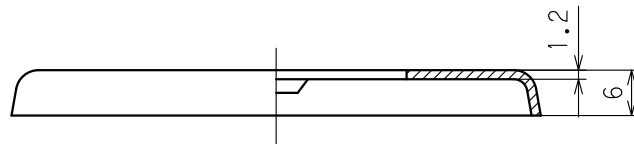
A-0-B断面図
