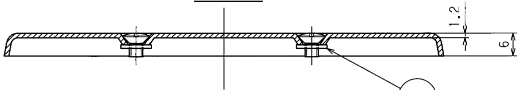
A-A'断面図
