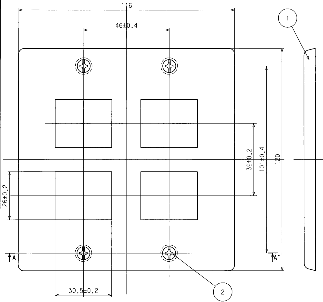
A-A'断面図
