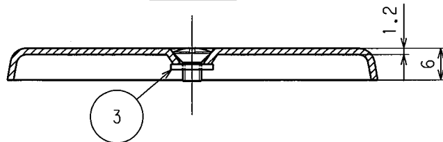
A-A' 断面図
