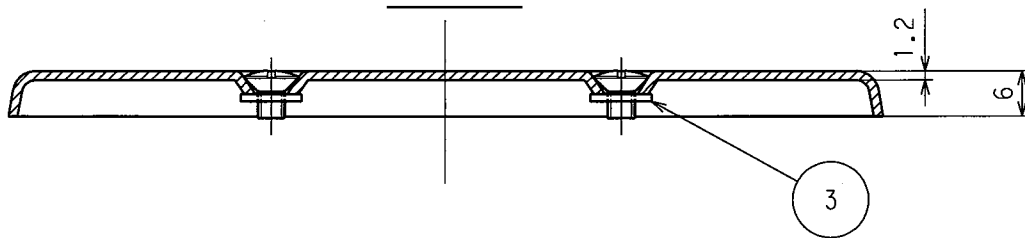
A-A'断面図
