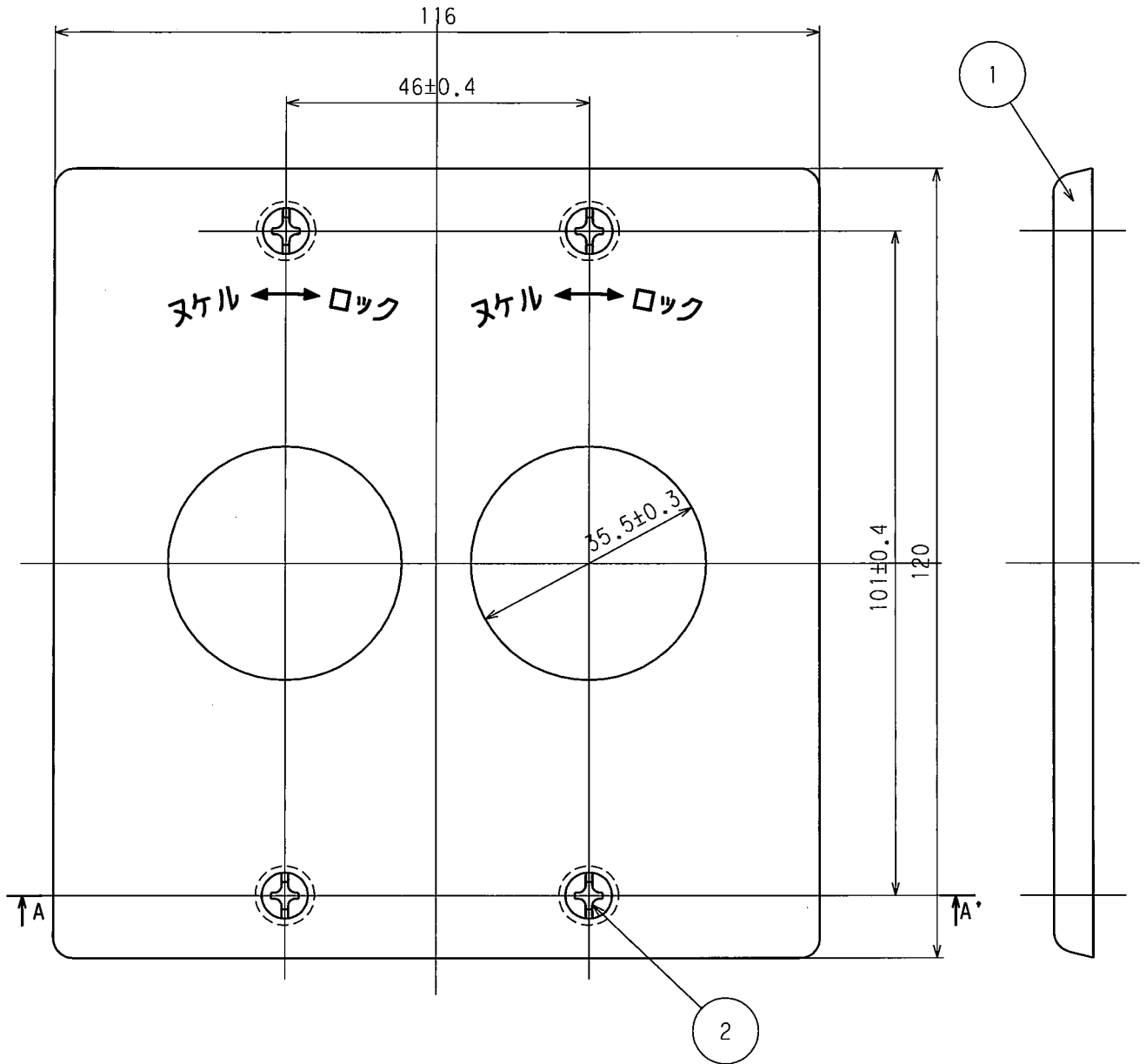
A-A'断面図
