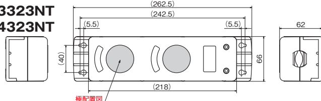
極配置図
