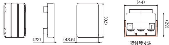
取付時寸法
