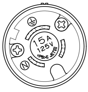
さし込みプラグ正面図
