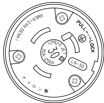
さし込みプラグ正面図
