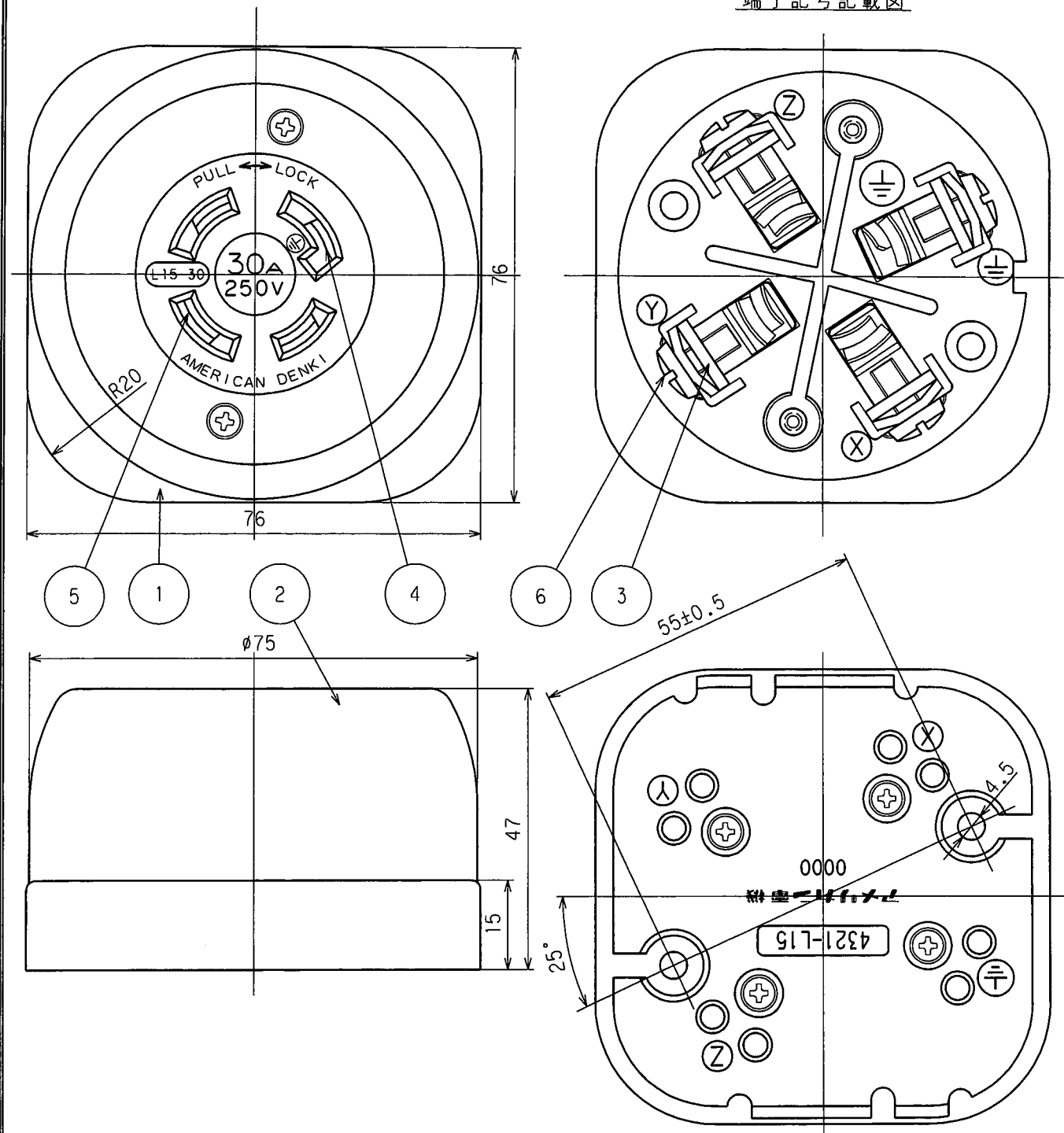
端子記号記載図
