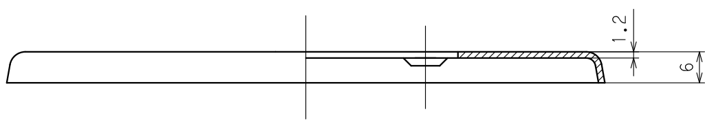
A-O-B断面図
