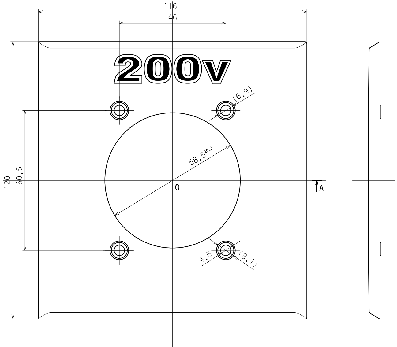
0-A断面図
