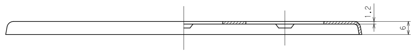
A-O-B断面図
