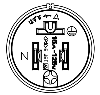
さし込みプラグ正面図
