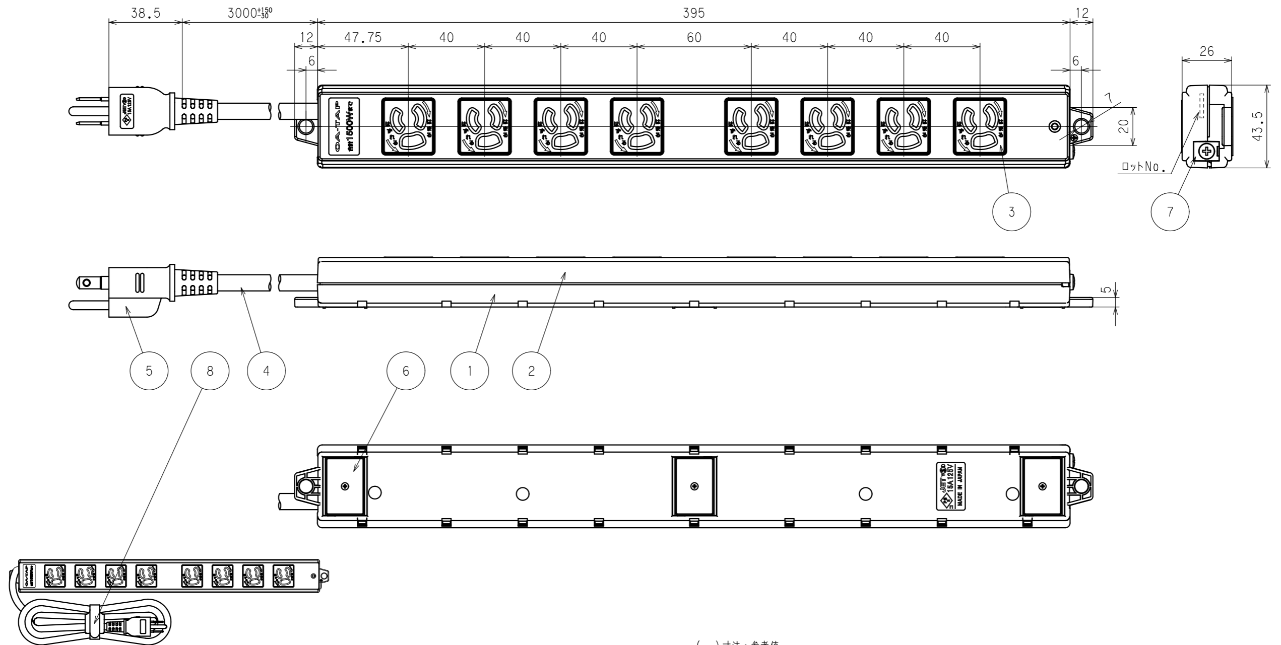
コード巻仕様
