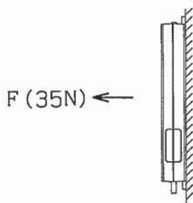
図1 マグネットの吸着力測定方法
