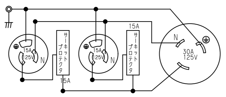
内部配線図
