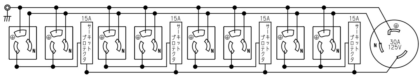
内部配線図
