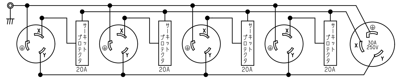
内部配線図
