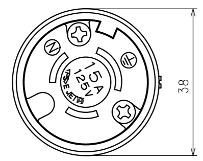
さし込みプラグ正面図
