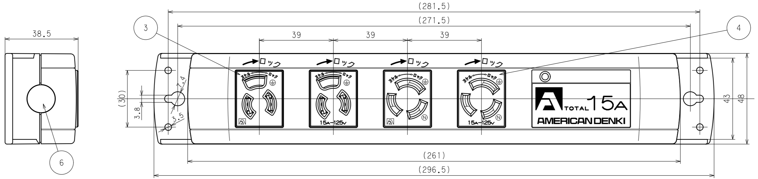
ブランクピース( 端末用フタ) 送り配線をする場合は、 取除いてご使用ください。
